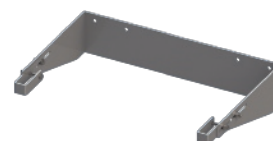
Wandbefestigung U-Form, zu Steigleiter ,verstellbar 275 - 375 mm
