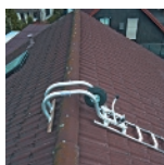
First-Überwurfbügel
