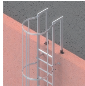
Ausstiegshilfen abgestützt zu Steigleiter
