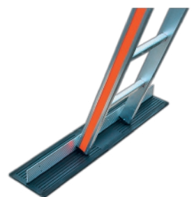
Antirutschmatte L 1270 x T 310 mm
