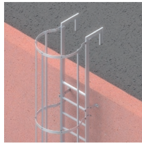
Ausstiegshilfen zu Steigleiter
