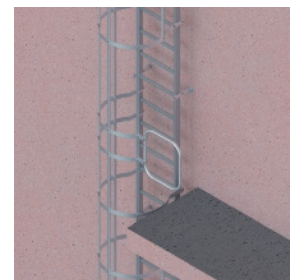
Selbstschliessende Türe zu Steigleiter für Seitenausstieg
